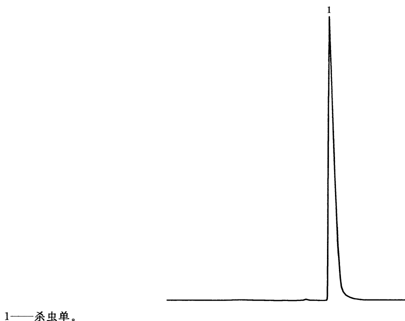
图 2 杀虫单原药的高效液相色谱图
